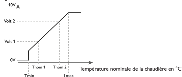
Signal de tension en V
