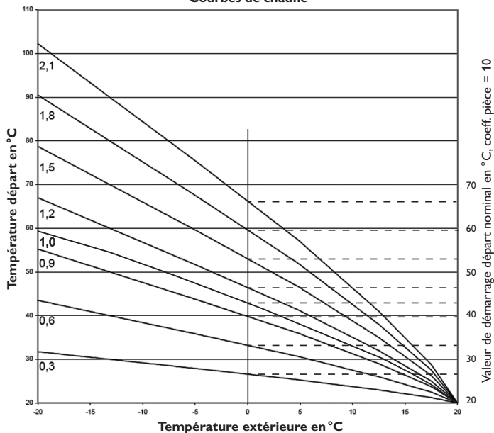
Courbes de chauffe
