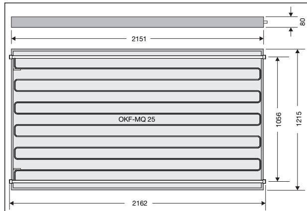
Abb. 6: Abmessungen
