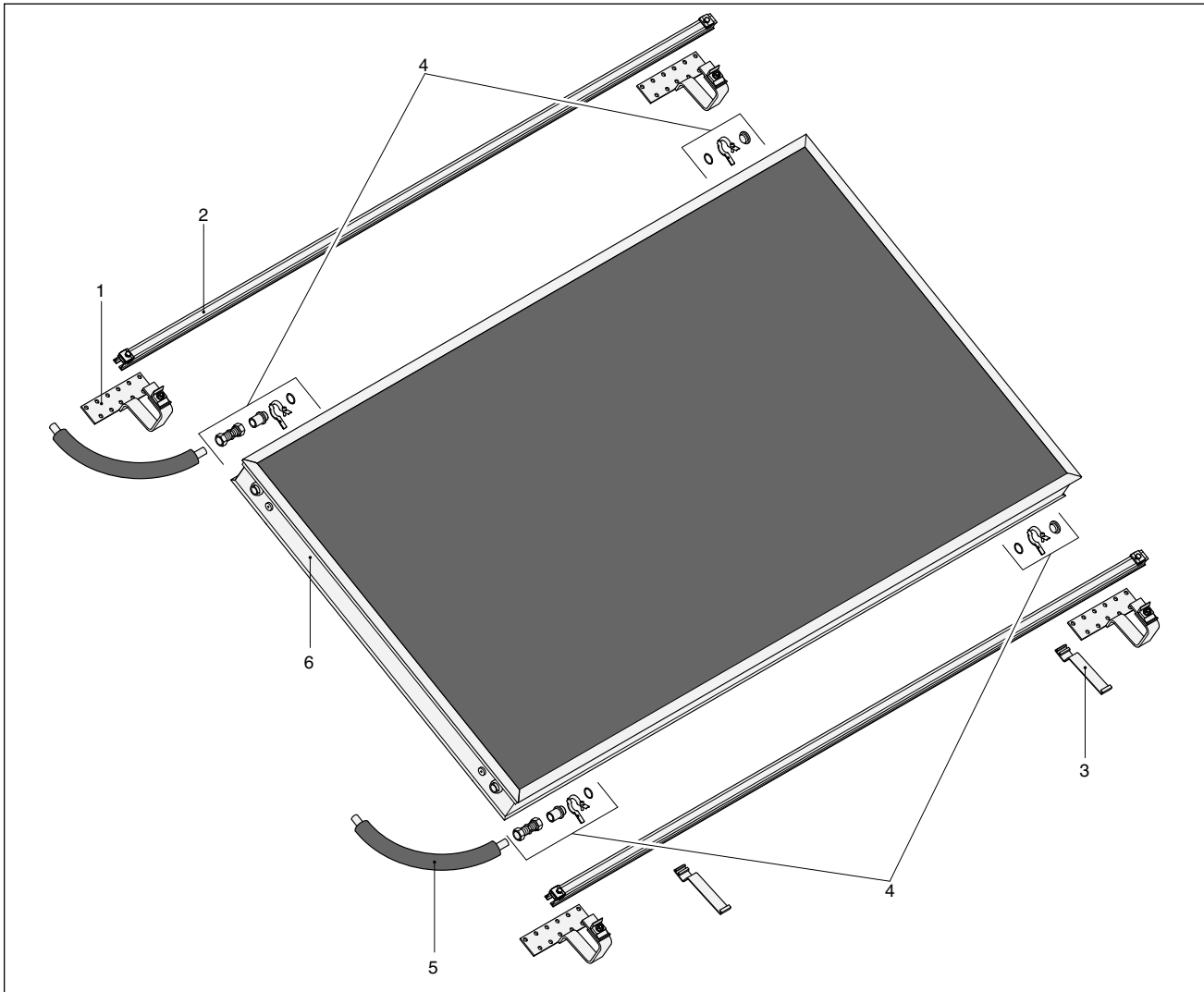
Abb. 10: Grundset Aufdachmontage
