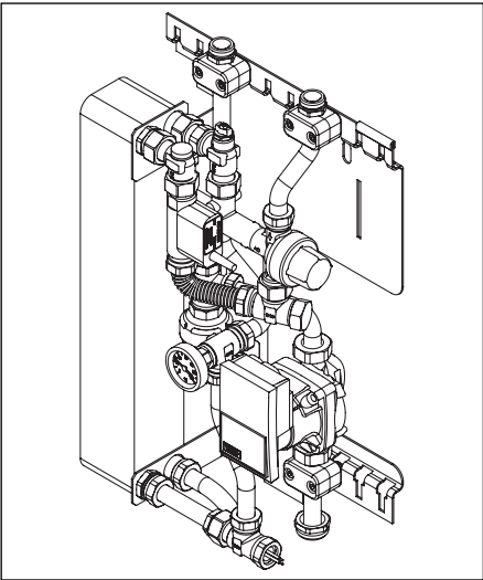
Abb. 24 Gesamtansicht „Regumaq XH“
