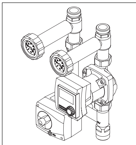
Abb. 20 „Regumat M3-130“ DN20
