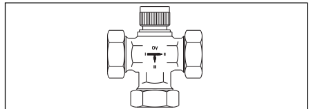
Abb. 39 Drei-Wege-Ventil für Zwei-Zonen-Beladung (113 02 06).
