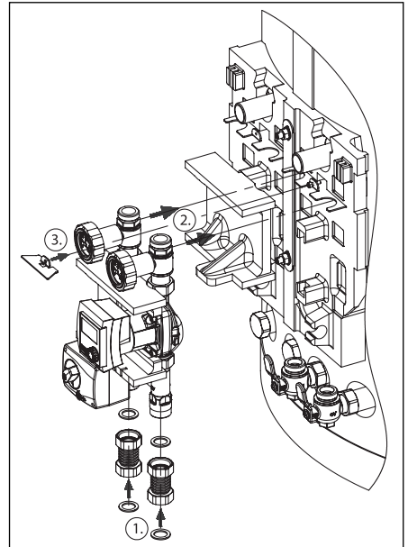
Abb. 10 Montage Heizkreisgruppe
