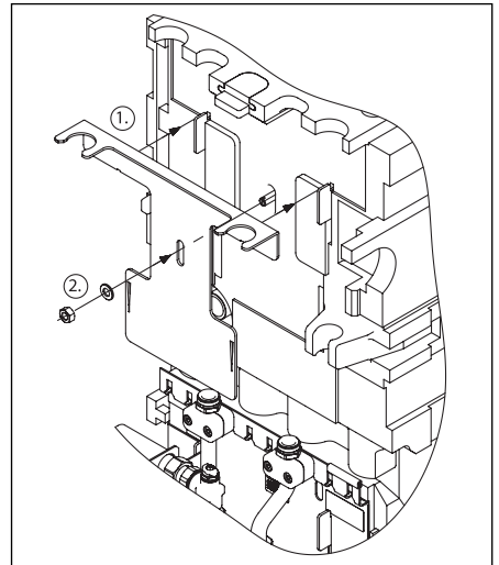
Abb. 17 Montage Solargruppenvorbereitung
