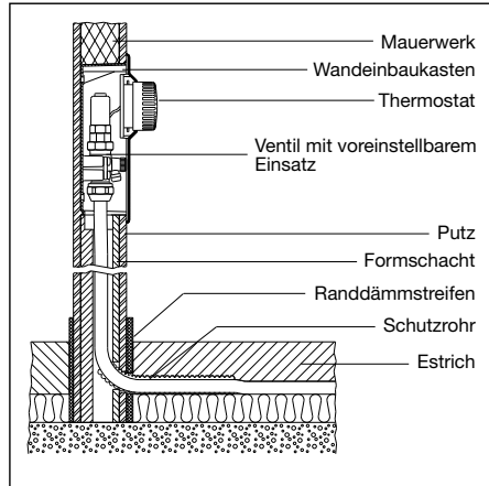
Schnitt
