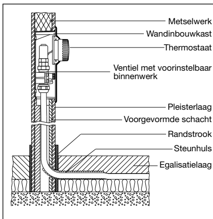
Inbouwplan
