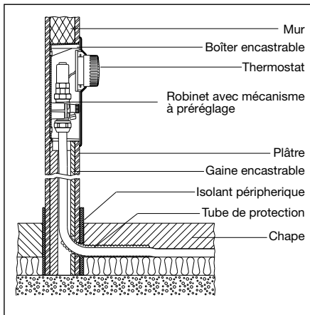
Coupe
