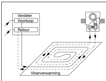
Inbouwplan
