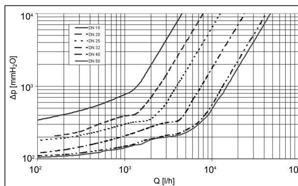
Diagrama pierderilor de presiune
