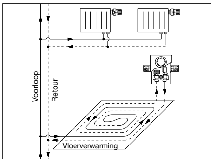
Inbouwplan
