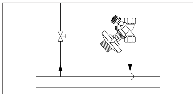
Příklad: Regulace průtoku např. v chladicích zařízeních. Přednastavení na regulátoru je nastavitelné a odečítatelné zvenku.
