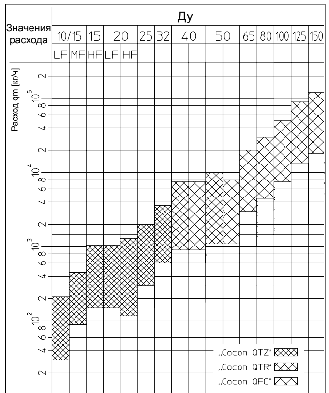
„Cocon QTZ/QFC“ с приводами
