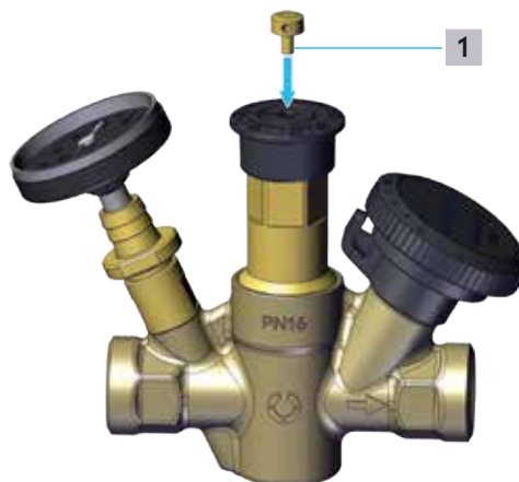
Fig. 9: Blocage de la valeur de consigne de température
