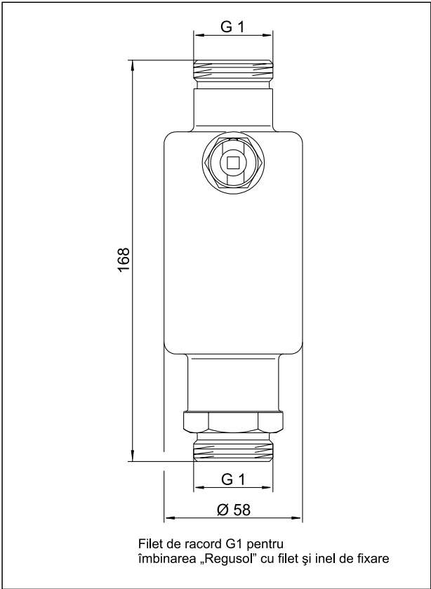
Vasul „Regusol” al dezaeratorului
