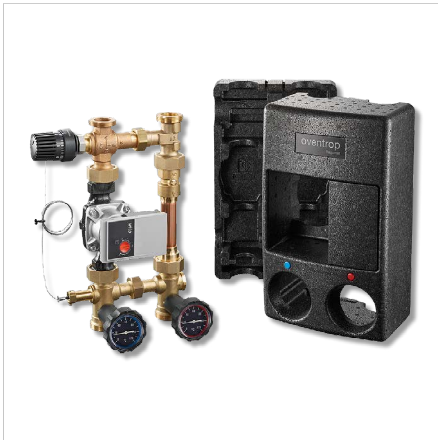
“Regumat RTA-180” DN 25 con bomba de alta eficiencia y aislamiento térmico universal
