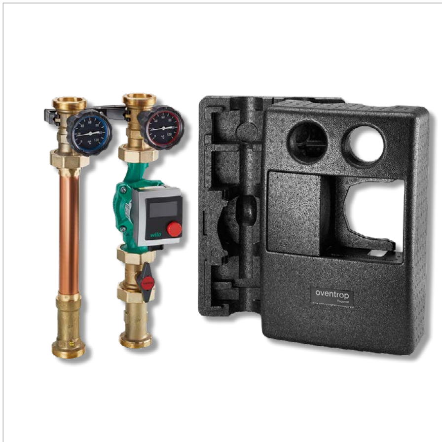
“Regumat S-180” DN 32 con válvula de bola de bomba a las entrada de la bomba de alta eficiencia
