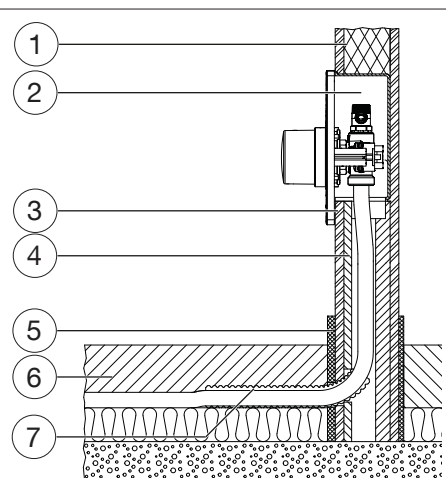
Abb. 9: Einbauquerschnitt
