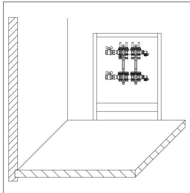
„Multidis“ Edelstahl-Verteiler im Einbauschrankschrank
