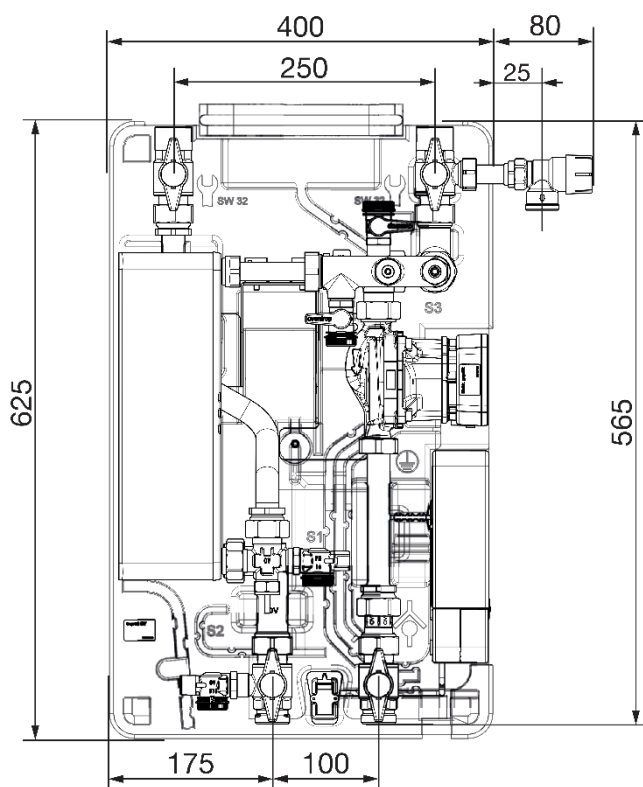
Afmetingen Regumaq X-45 (voorkant)
