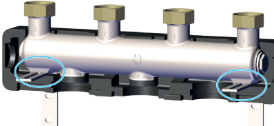
Fig. 6: Fixation du bloc de répartition sur les supports muraux
