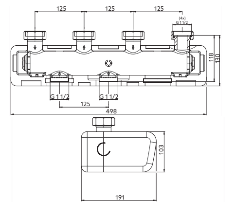
Fig. 2: Encombrements
