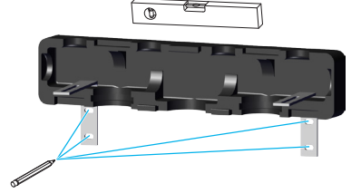
Fig. 5: Marquage des trous de perçage
