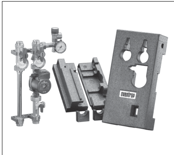
„Regusol”-overgangstation
