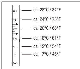
Abb. 5 Temperaturskala Thermostat „Uni LH“
