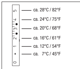
Obr. 5 Teplotní stupnice termostatické hlavice „Uni LH“
