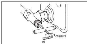
Fig.3 Intercettazione del detentore a servizio del radiatore
