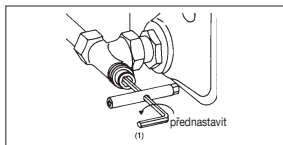
Obr. 4 Nastavení šroubení
