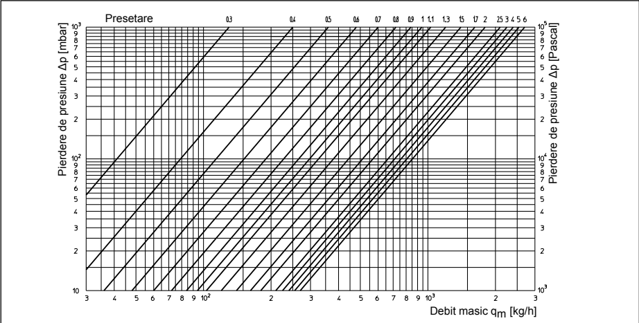
Diagrama 7.2: Pierdere de presiune ventil de echilibrare „Hycocn VTZ“ DN 20
