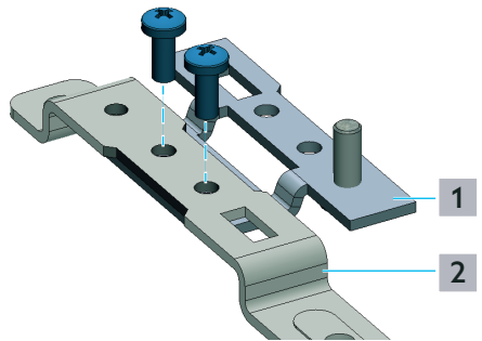
1 Dispositif de compensation de montage pour distributeurs/collecteurs pour circuits de chauffage Multidis
