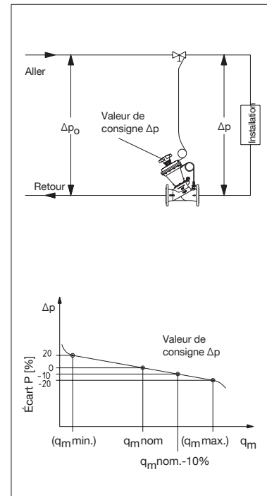
Schéma d'installation
