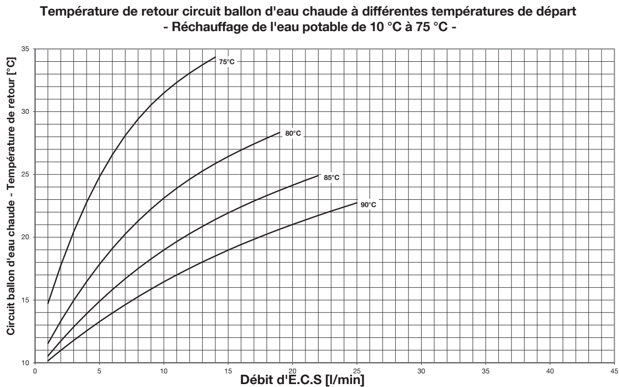
Fig. 55: Température de retour du circuit ballon d'eau chaude - Réchauffage de l'eau potable à 75 °C
