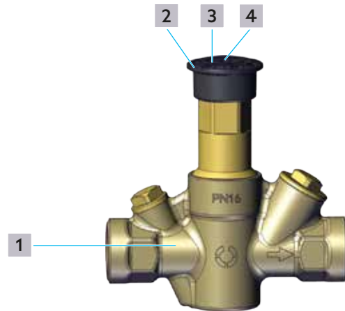
Abb. 1: Aufbau
