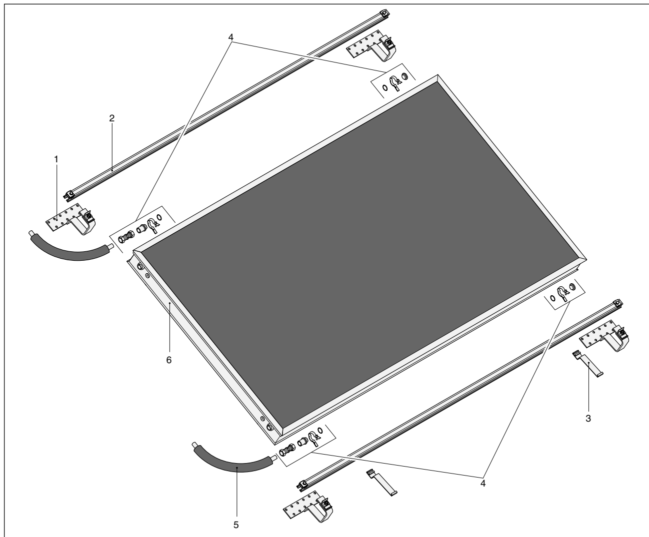
Abb. 10: Grundset Aufdachmontage
