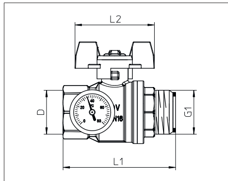
Abb. 6: Maße Kugelhahn
