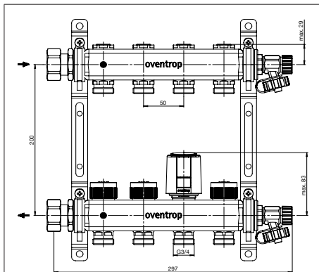
Abb. 5: Maße
