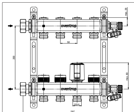
Рис.5: Размеры
