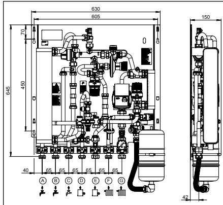
Abb. 4.1 Abmessungen
