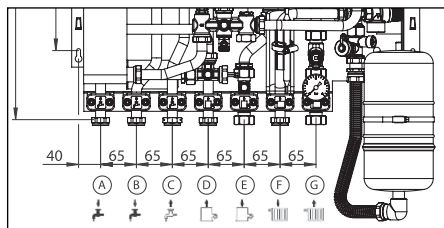
Fig. 4.2 Collegamenti
