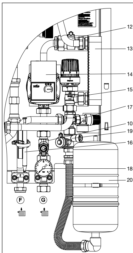
Fig. 8.3 Remplissage
