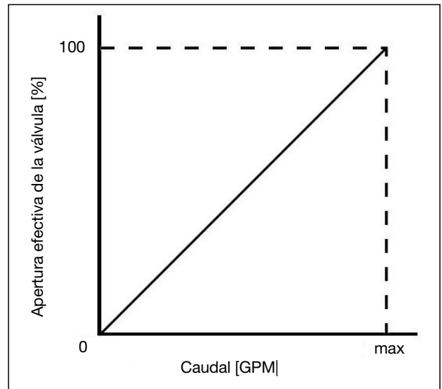
Figura 9 Curva característica de la válvula “Cocon QFC/QGC”
