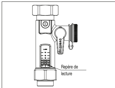
Fig. 4.5 Robinet d'équilibrage
