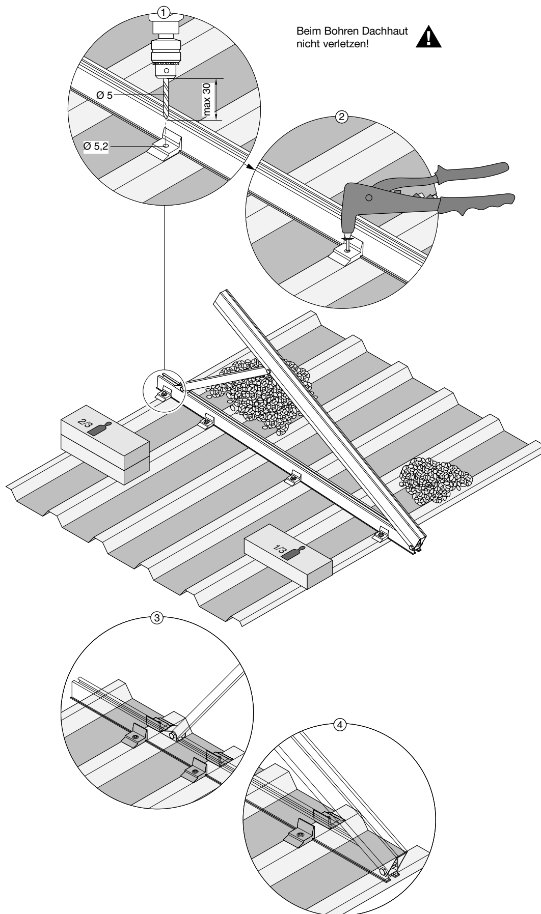
Abb. 27: Befestigung der Aufstelldreiecke: Bodenschiene im Bereich der Stützschiene beidseitig mit 4 Klemmwinkeln einfassen (3). Im vorderen Bereich (4) beidseitig mit 2 Klemmwinkeln befestigen.
