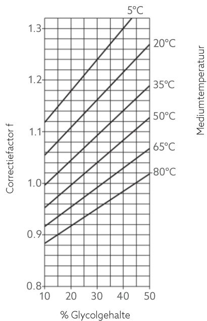
Correctiefactor f - ethyleenglycol
