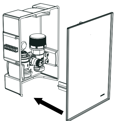
Abb. 10: Abdeckung aufsetzen
