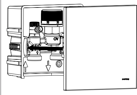
Abb. 7: Abdeckung aufsetzen
