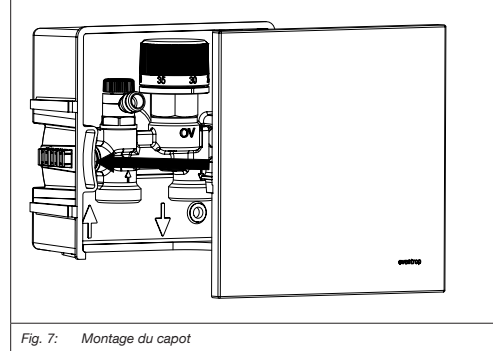
Fig. 7: Montage du capot
