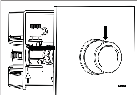
Abb. 6: Abdeckung mit Handrad aufsetzen
