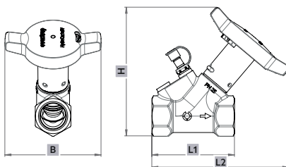
Obr. 2: Rozmery, náhľad z boku/náhľad spredu, vnútorný závit
