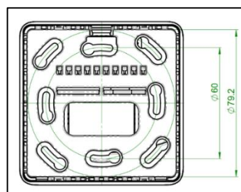
Maße Montageplatte ClimaCon
