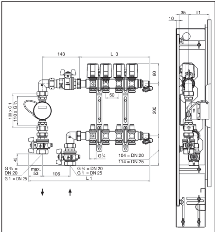
Abb. 2 Beispiel: Wärmemengenzähler-Anschluss-Set, Eckform und „Multidis SFQ“ Edelstahl-Verteiler für Flächenheizung und -kühlung, Baulängen und Bautiefe
