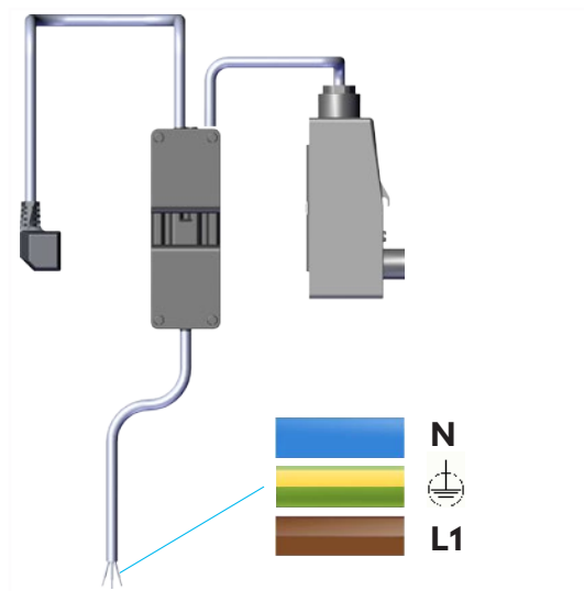
Abb. 7: Adernbelegung
