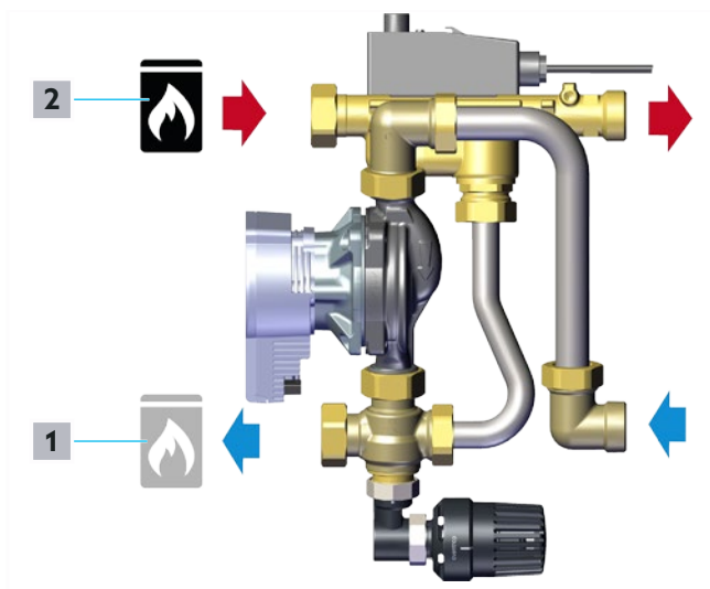
Abb. 5: Durchflussrichtung
