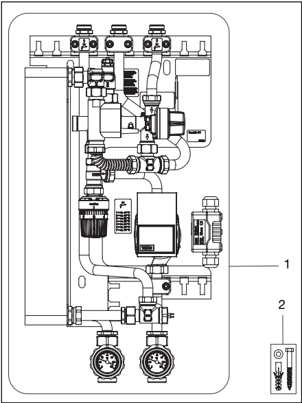
Abb. 3.1 Lieferumfang
