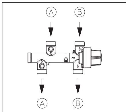
Abb. 5.4: Proportional-Mengenregler
