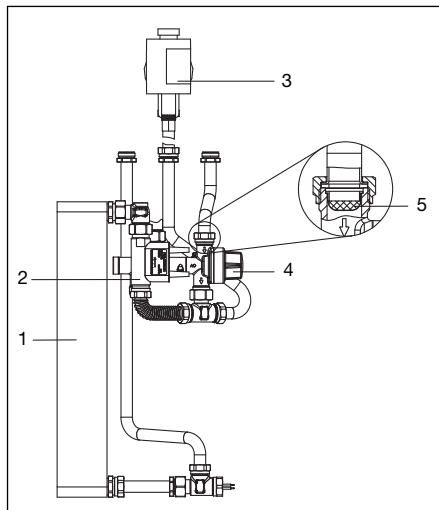
Abb. 5.3: Sekundärkreislauf
