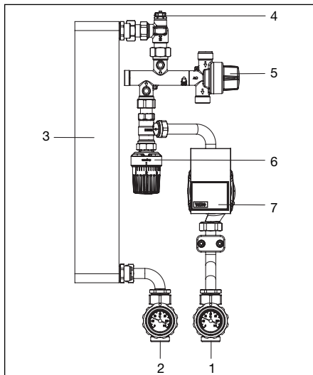
Abb. 5.2: Primärkreislauf
