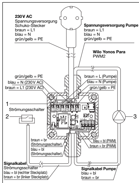
Abb. 6.6: Verkabelung Primärkreis
