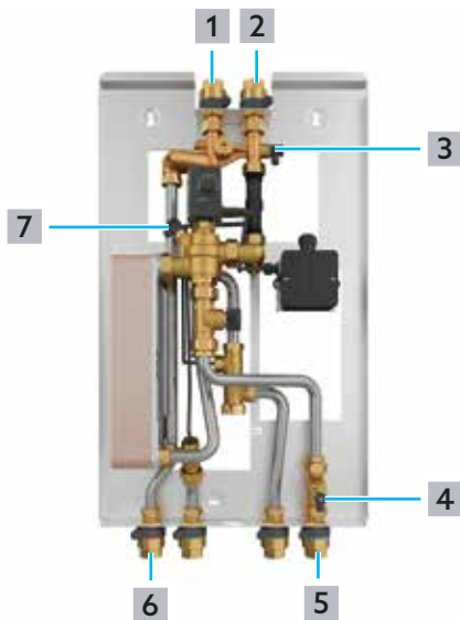
Abb. 14: Heizkreis füllen und entlüften
