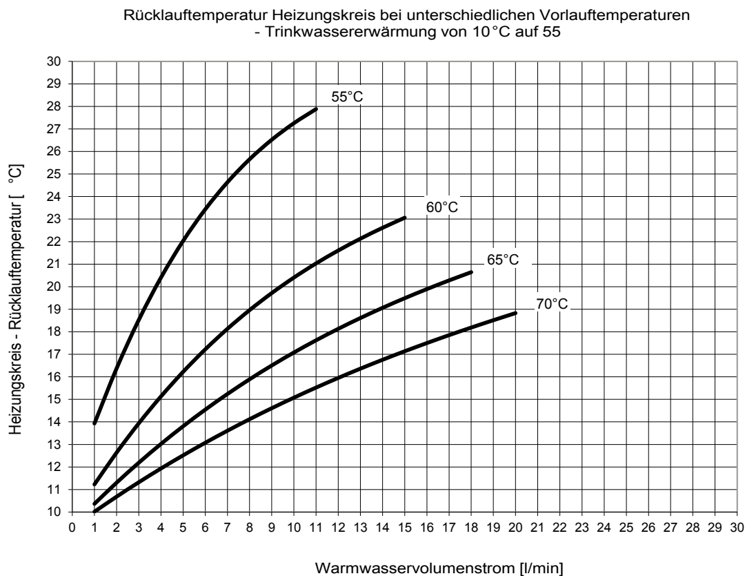
Abb. 37: Leistungsbereich 1, Trinkwassererwärmung auf 55 °C
