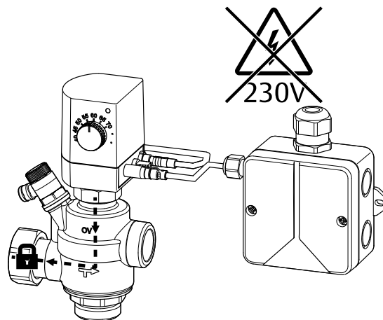
Abb. 2: Regelventil schließt bei Stromausfall
