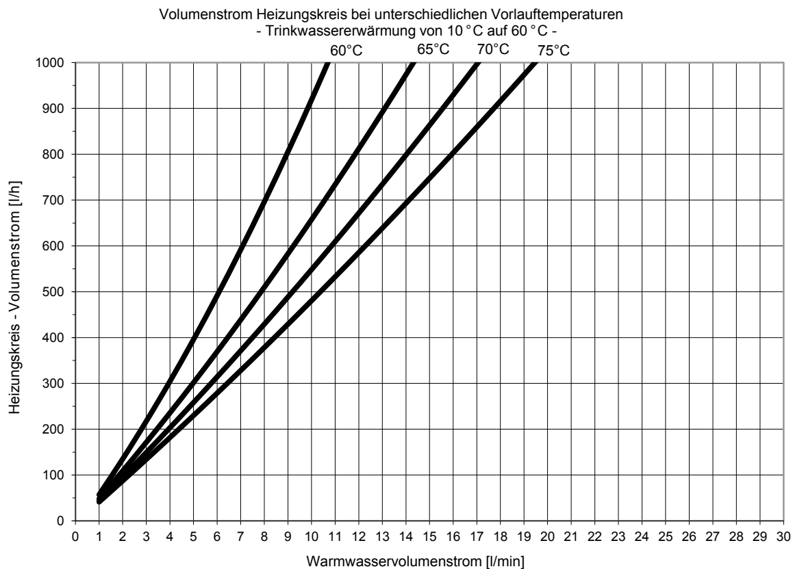
Abb. 38: Leistungsbereich 1, Trinkwassererwärmung auf 60 °C
