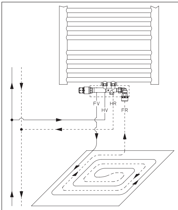
Schéma d'installation
