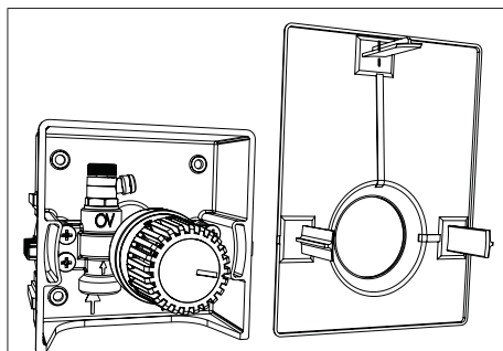
Abb. 18: Rückseite Abdeckung
