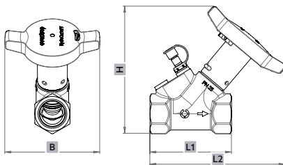
图 2: 内螺纹款侧视图/正视图尺寸
