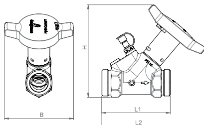
Bild 3: Mått sidovy yttergänga
