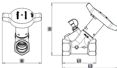
Fig. 2: Dimensiones vista lateral / vista frontal rosca interior
