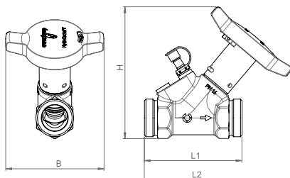
Afb. 3: Afmetingen zijaanzicht buitenschroefdraad
