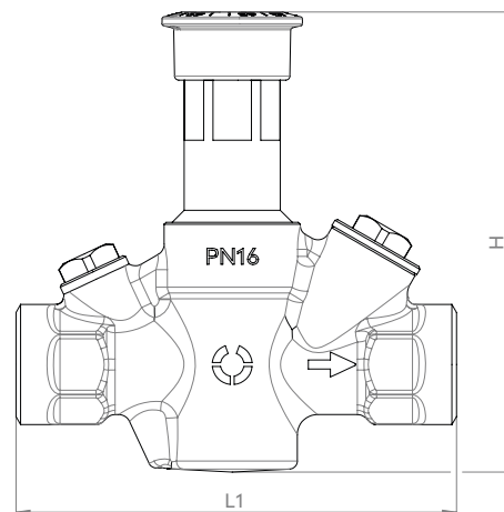
Fig. 2 - Dimensioni della parte laterale
