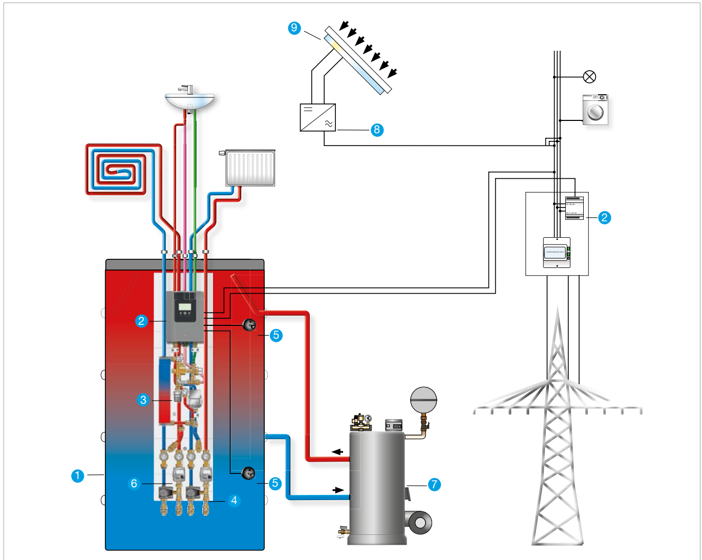
System-Darstellung „Regucor WHP“ in Verbindung mit konventionellem Wärmeerzeuger
