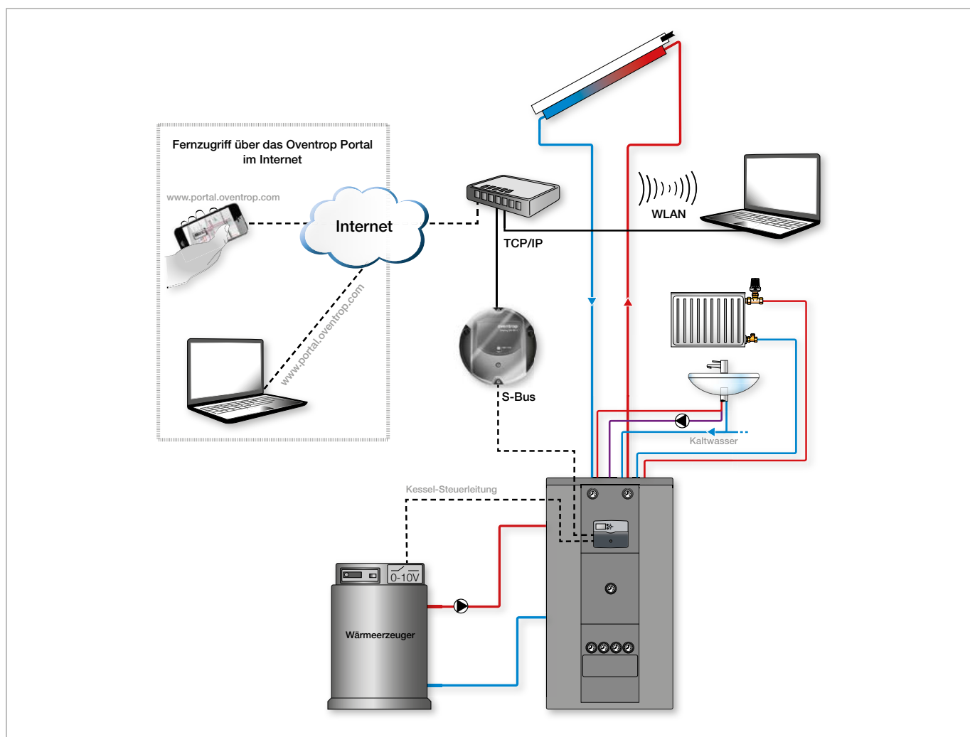
System-Darstellung „Regucor WHS“ Energiespeicher-Zentrale für Solarthermie, Trinkwasser und Heizung
