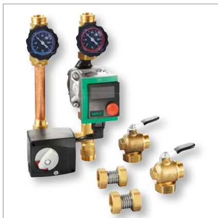
Anbaugruppe Heizkreis
