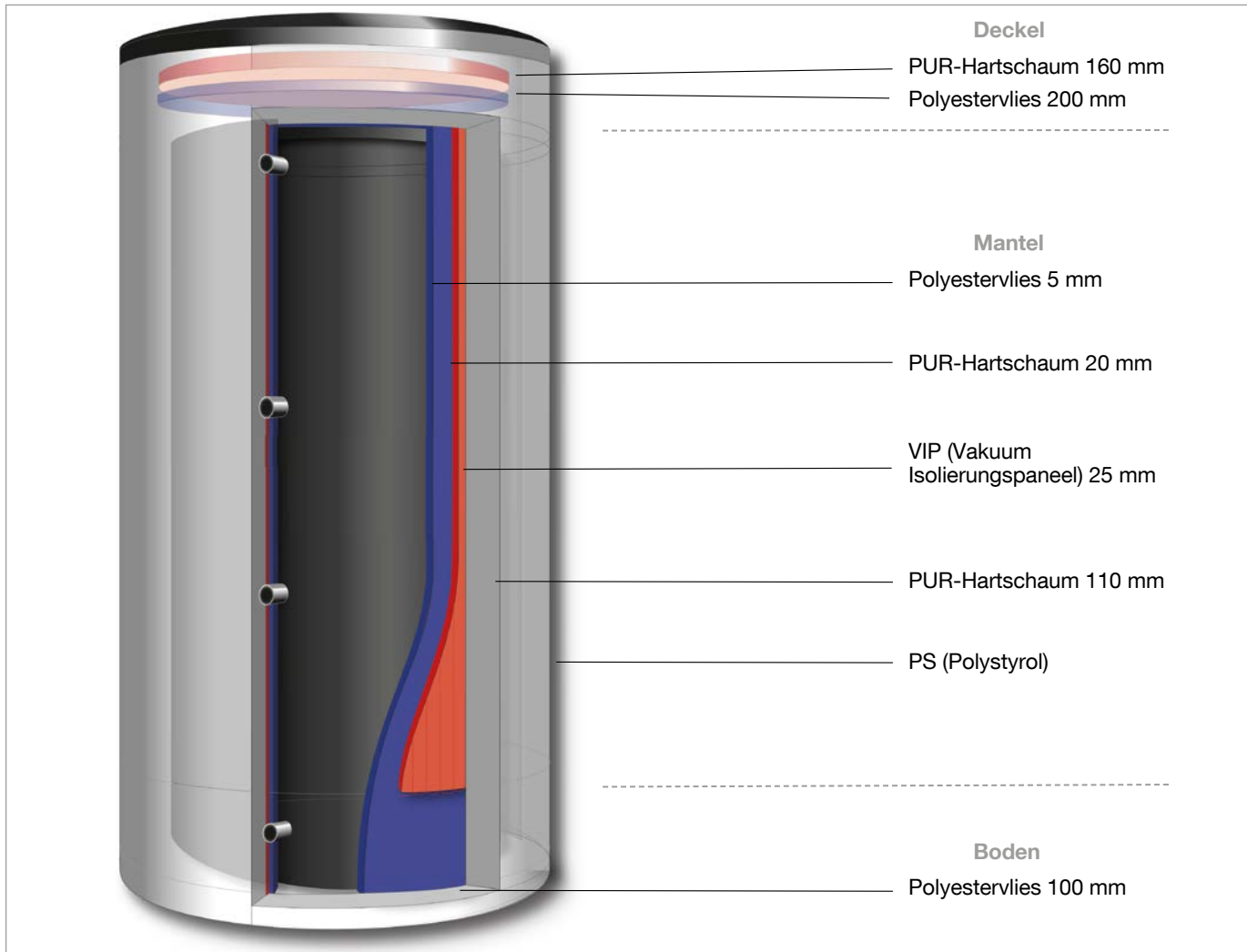
Schichtaufbau der Isolierung des „Regucor WHS“, Typ 500, Energieeffizienzklasse A
