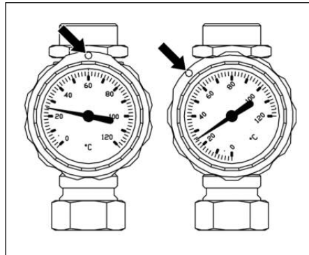
Abb. 20: Kugelhahn Speichervorlauf
