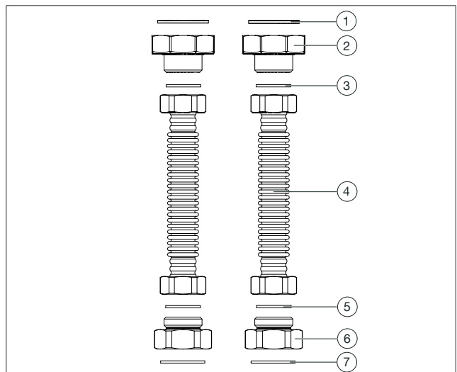
Abb. 29: Aufbau Verbindungsset
