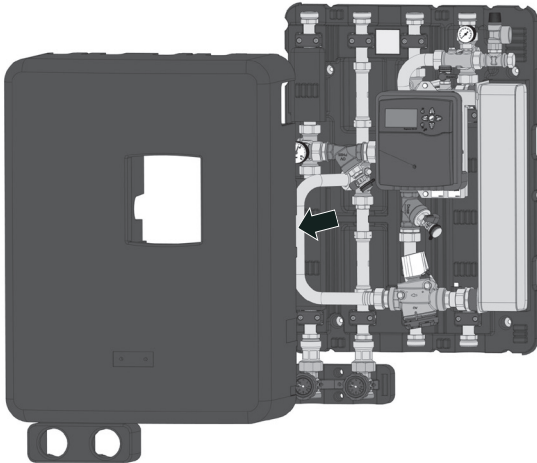
Abb. 26: Wärmedämmoberschalen entfernen
