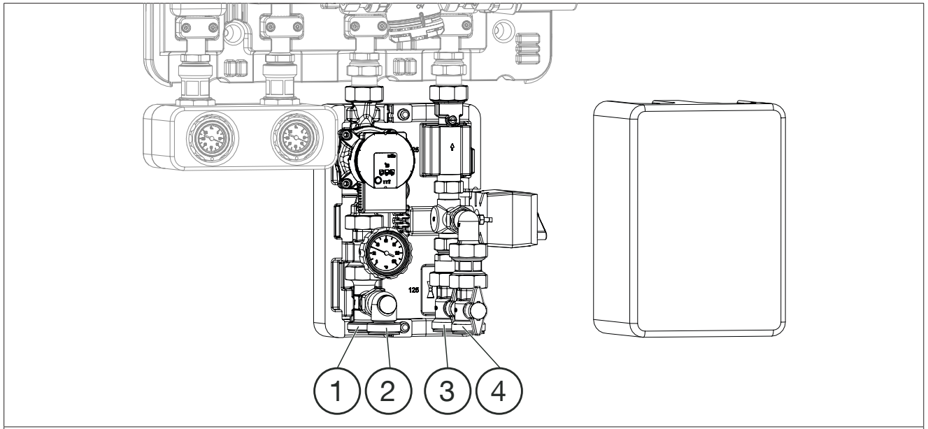
Abb. 12: Anschlüsse HT-Umschaltmodul
