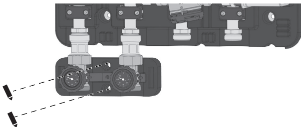
Abb. 27: Bohrlocher Befestigungsschrauben markieren
