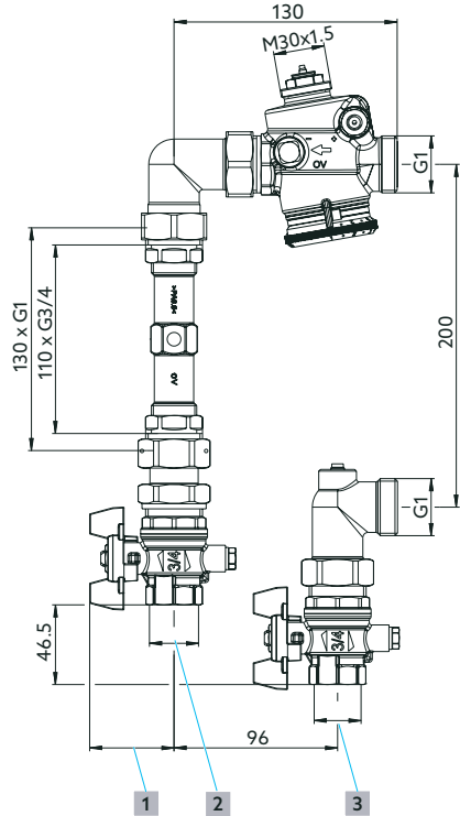
Abb. 3: Abmessungen Eckausführung
