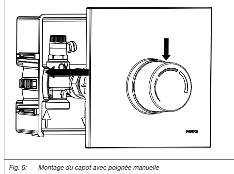
Fig. 6: Montage du capot avec poignée manuelle
