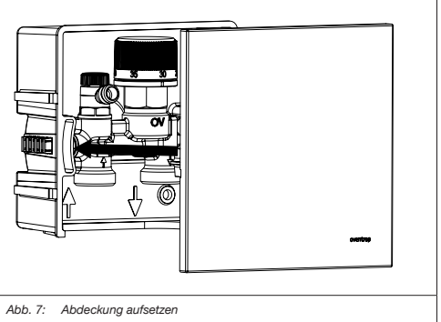
Abb. 7: Abdeckung aufsetzen
