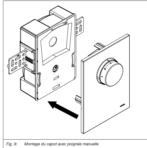
Fig. 9: Montage du capot avec poignée manuelle
