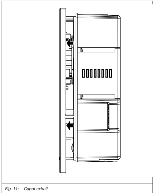
Fig. 11: Capot extrait
