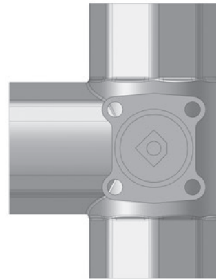
Abb. 3.17: Rückschichtkugelhahn, Art.-Nr. 1381192-94
