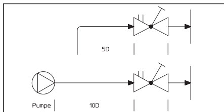
Abb. 4 Einbauhinweise
