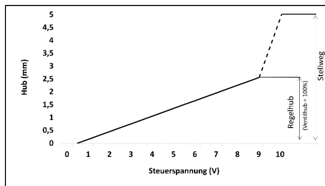
Hub-Steuerspannungs-Kennlinie bei erkanntem Ventilweg
