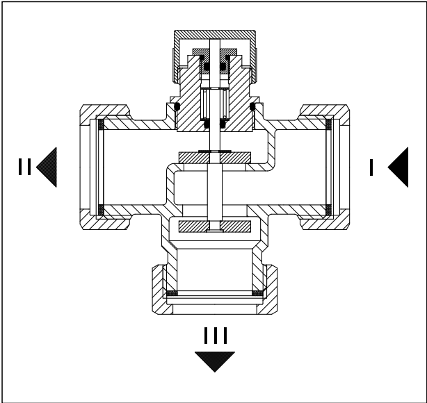
Schnittbild
